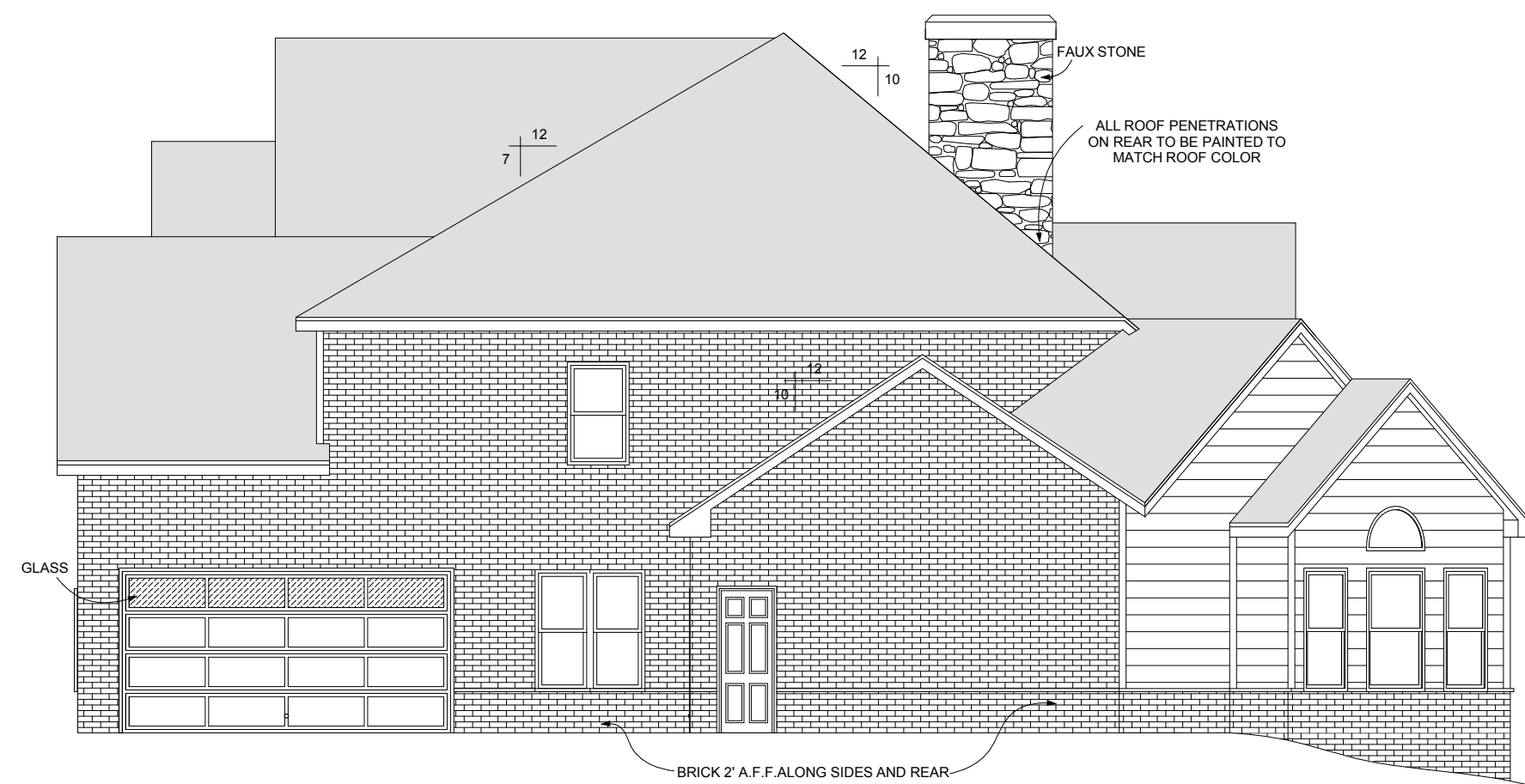
RIGHT ELEVATION
